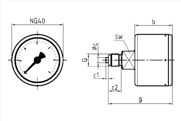
Maße (mm)
