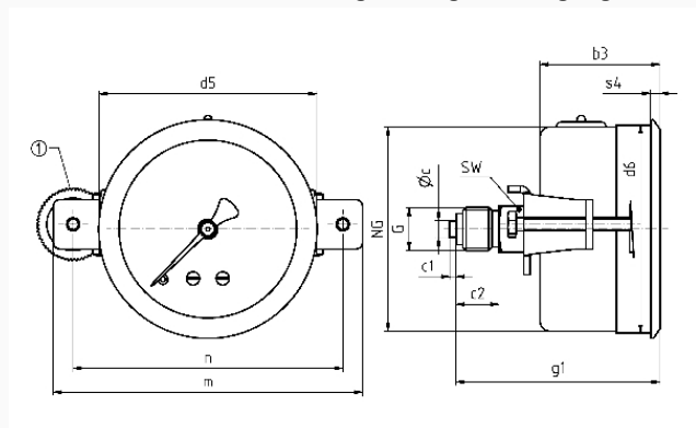
Anschluss axial, 3-Kantfrontring mit Bügelbefestigung
