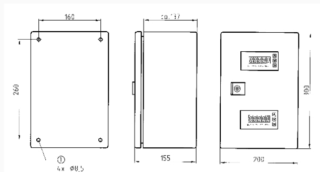
Wandaufbaugehäuse WAG 01/02 zur Aufnahme von max. 2 DA 10/12/14
