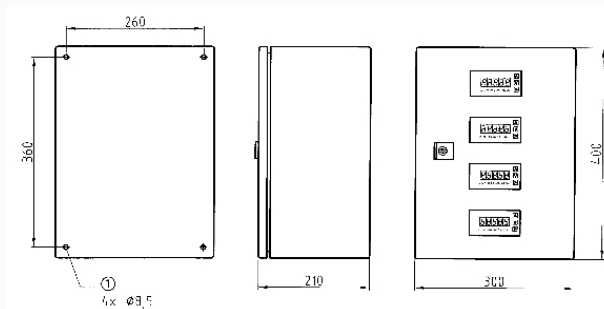
Wandaufbaugehäuse WAG 03/04 zur Aufnahme von max. 4 DA 10/12/14
