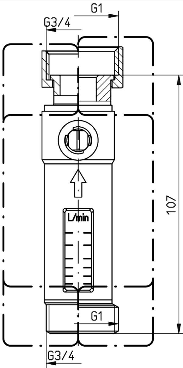
DFM 15-2M, Aussengewinde x Überwurfmutter
