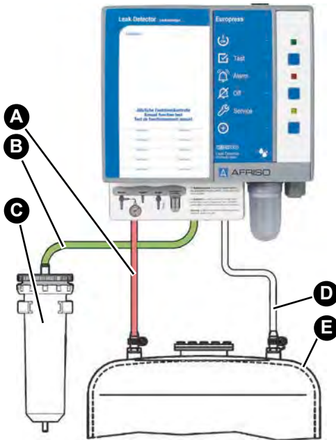
Figure 2: Branchement d'un réservoir aérien
