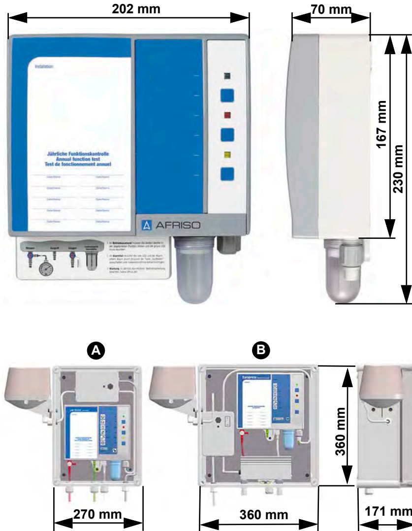
Afbeelding 1: Europress in beschermende behuizing, zonder (A) of met verwarming (B), aansluitklaar vooraf gemonteerd. De signaalhoorn is op het uitgangsrelais aangesloten.
