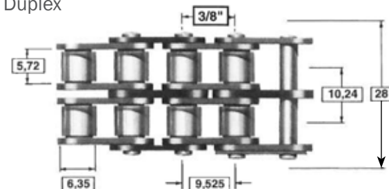
Duplex
