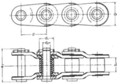
Utførelse A, DIN 8188
