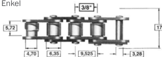
Enkel
