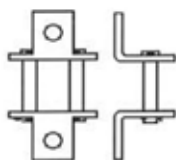
Bæreledd 170, 176 (K1) 172, 178 (K1)
