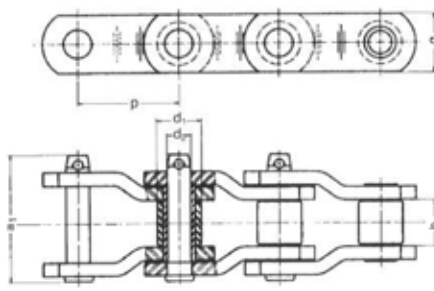
Utførelse B, DIN 8182
