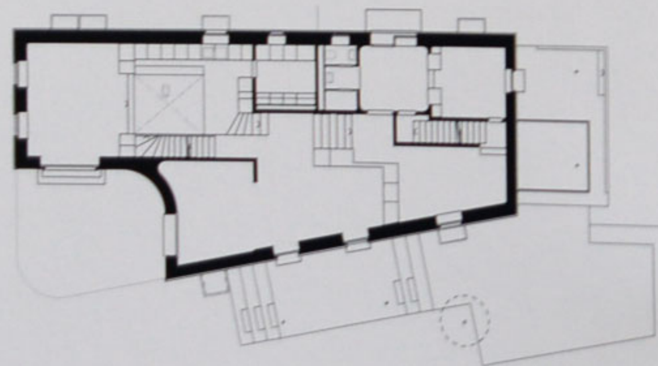
Erdgeschoss
