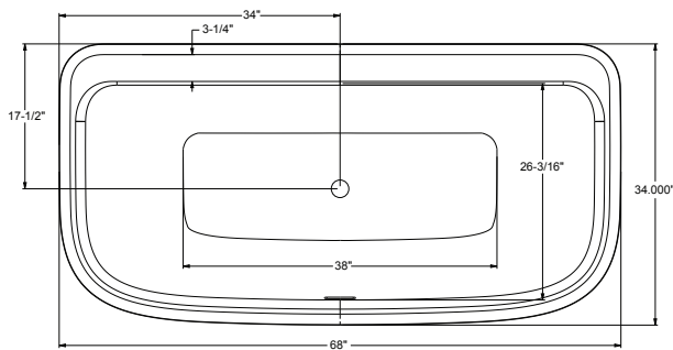
Tina interna
