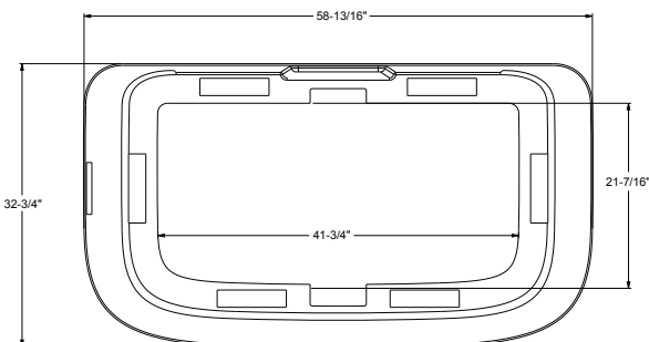
Cubierta exterior
