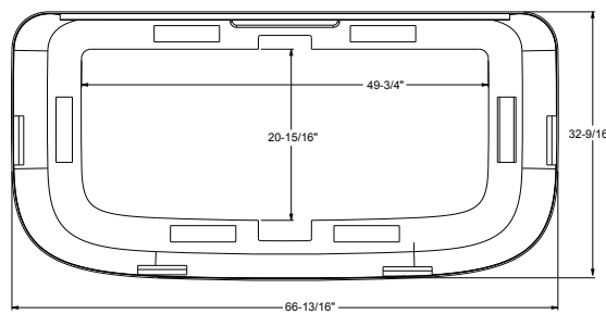
Cubierta exterior
