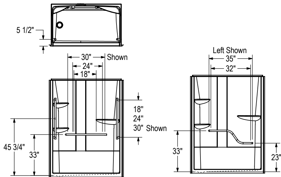
GRAB BAR Left Shown
