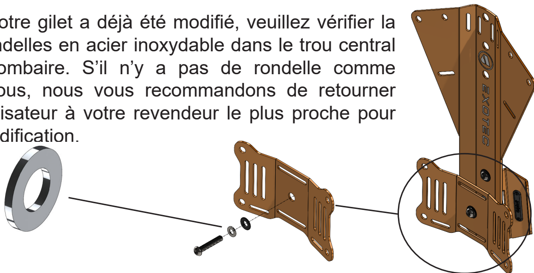
Rondelle inox
