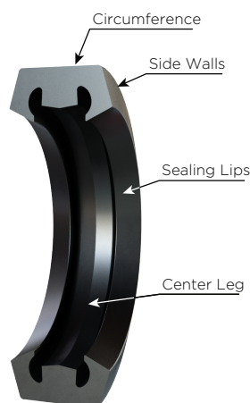
GapSeal Gasket
