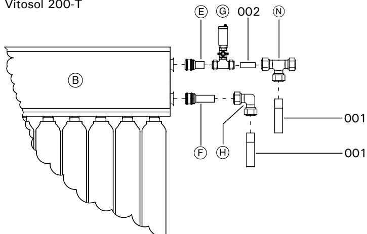
Vitosol 300-T
