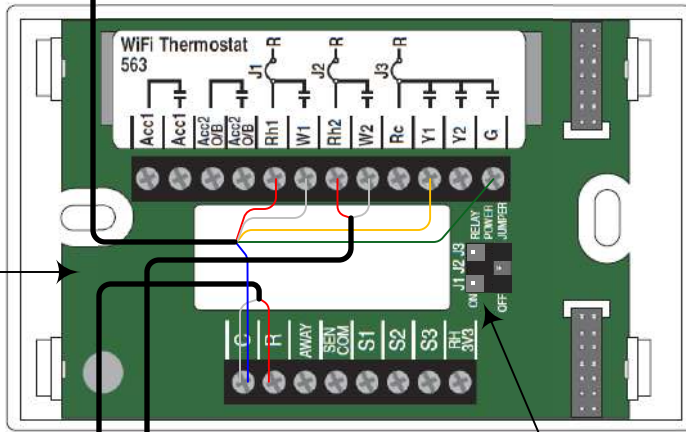
Tekmar 563 Wi-Fi T-stat
