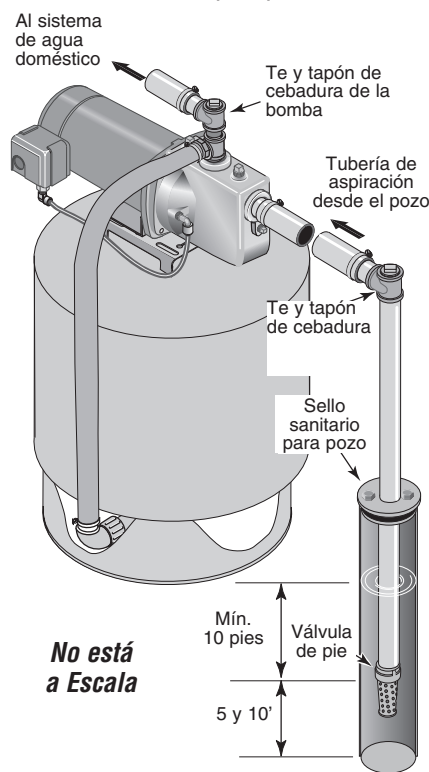
Figura 2: Instalación en pozo entubado
