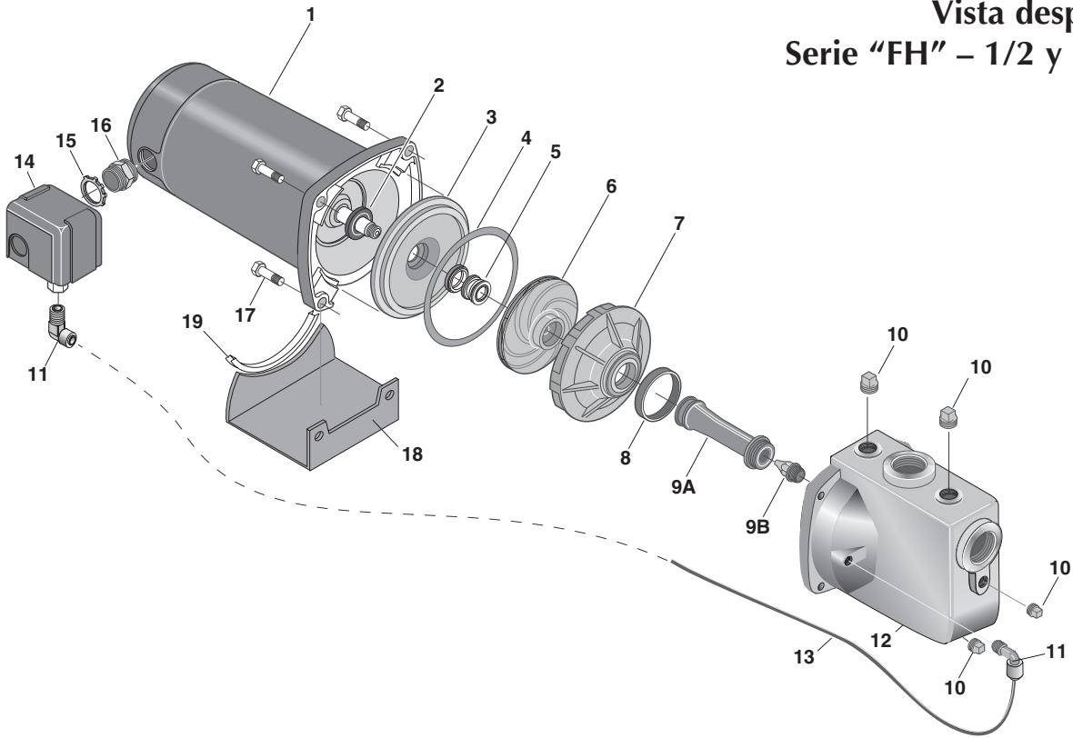
LISTA DE REFACCIONES: Serie "FH", 1/2 y 3/4 HP
