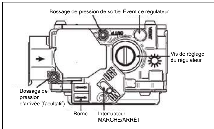
FIG. 28. - SOUPE DE GAZ WHITE RODGERS 36J24-214 (W010-2614)
