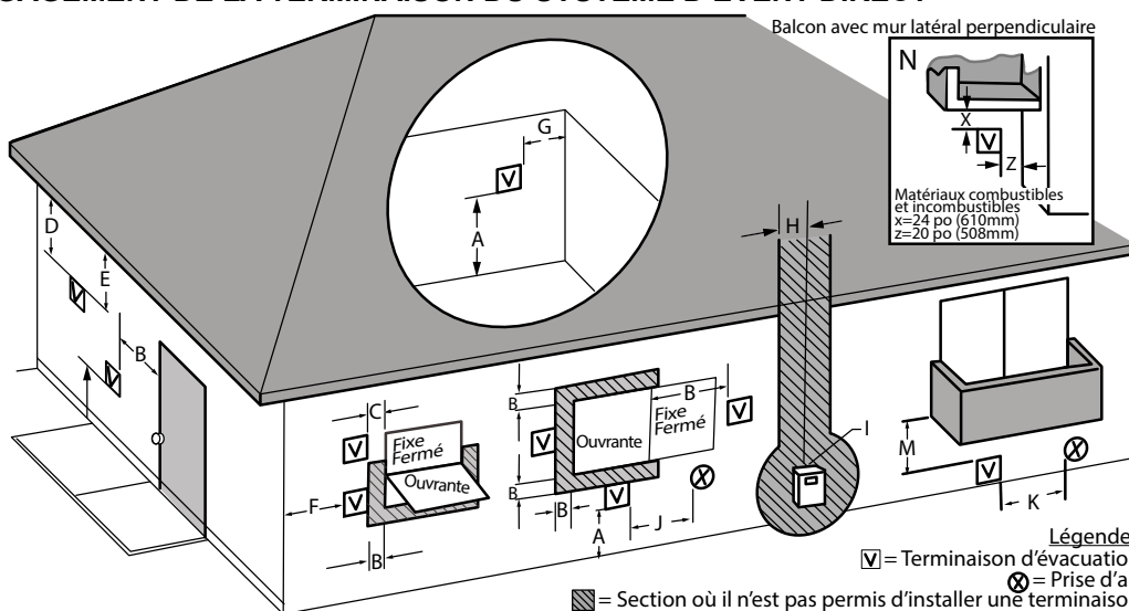
Balcon avec mur latéral perpendiculaire
