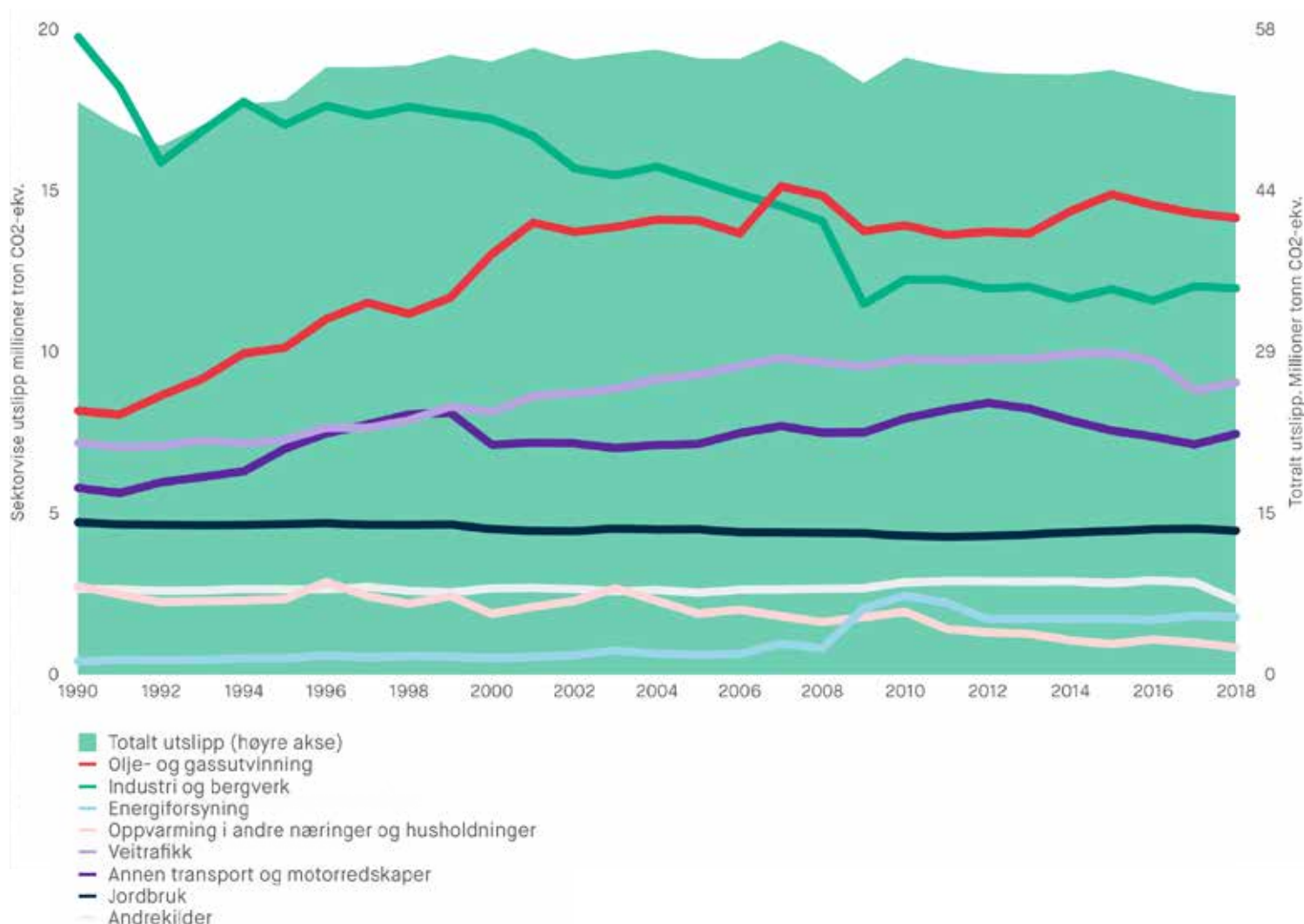
Utslipp av klimagasser totalt og sektorvis. 1990-2018. Kilde: SSB, som gjengitt i Statsbudsjettet.
