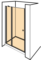
Nisopstelling = draaideur met vast paneel + muurprofiel
