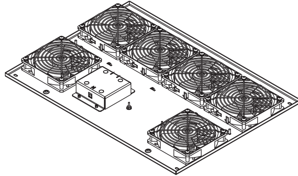
ERK-414FT-K-EU Fan Top
