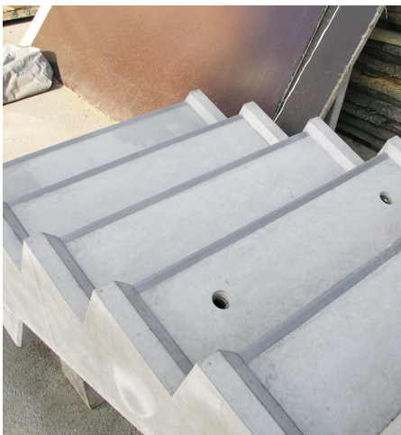
Fertigtreppe
