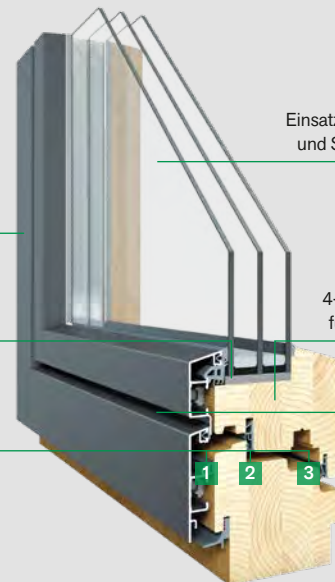
Festverglasung aus Holz mit Aluschale in Anthrazit
