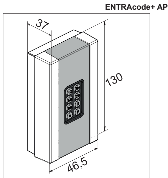
Abb. Abmessungen ENTRAcodes+ AP (alle Angaben in mm)
