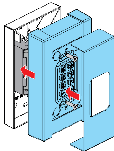
F. In umgekehrter Reihenfolge zusammenbauen.
