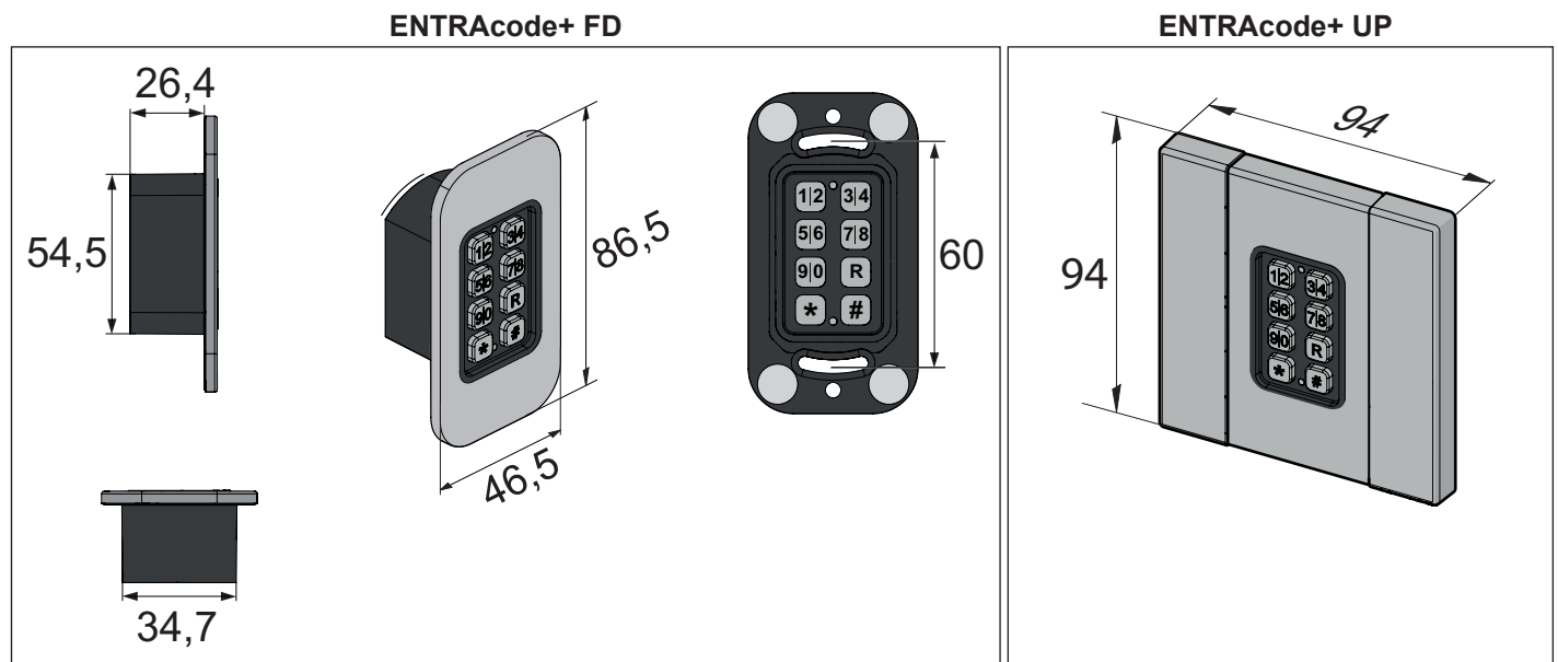
Abb. Abmessungen ENTRAcodes+ FD / UP (alle Angaben in mm)
