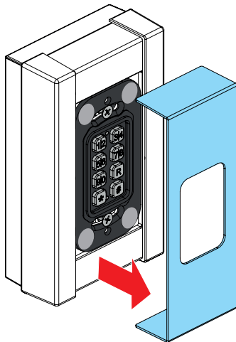
A. Magnetische Blende entfernen.
