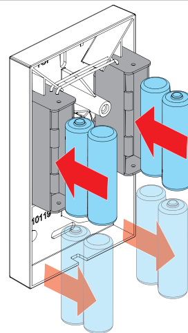
D. Alte Batterien entfernen.
