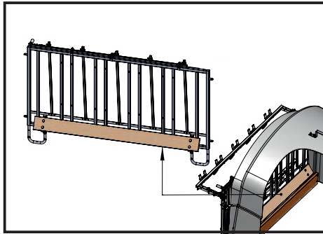
Trittschutzset #14529
