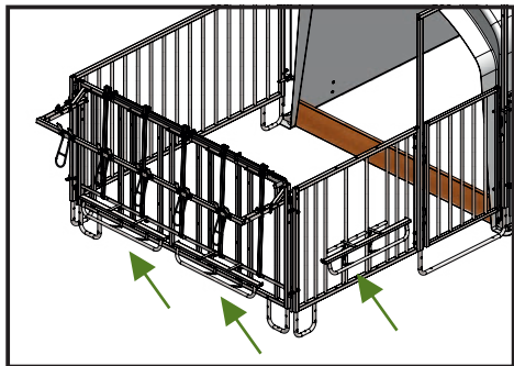
Troghalter für Langfüttertrog #14526
