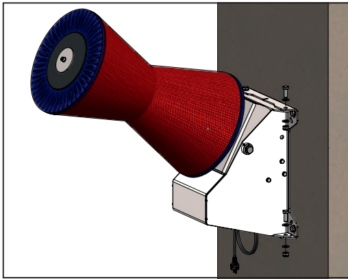
Abbildung 4: Verschraubung links oder rechts lösen
