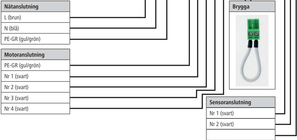
Bild 7: Kopplingsschema för krets-kortet med kondensator - Uno
