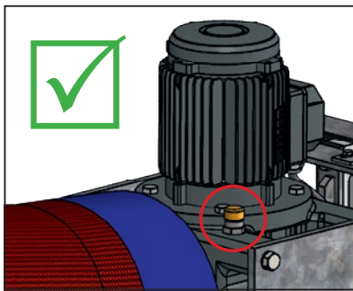
Kuva 4: Ilmausruuvien asennus
