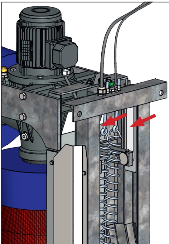
Abbildung 11 – Position Gleitführungen
