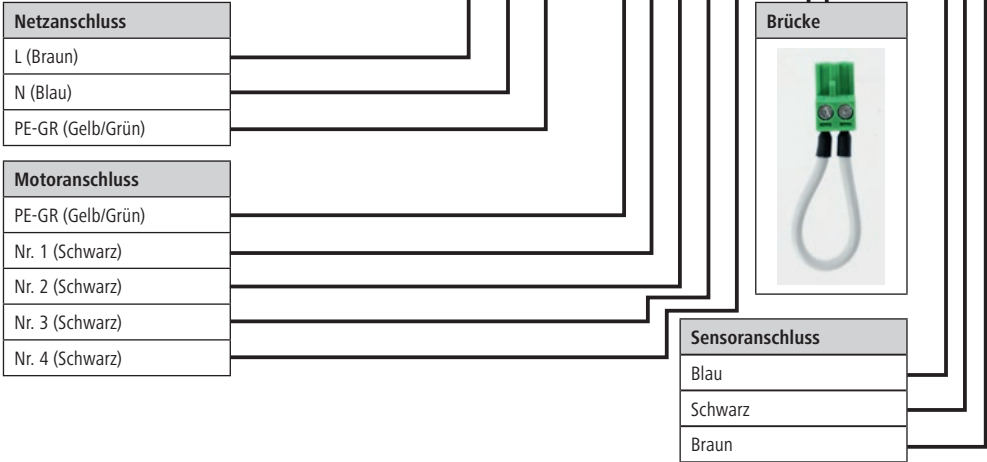
Abbildung 8: Anschlusschema der Platine mit Kondensator - Duo
