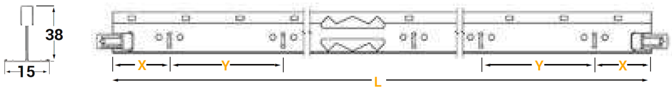
Tragschiene
