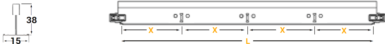
Querschiene kurz
