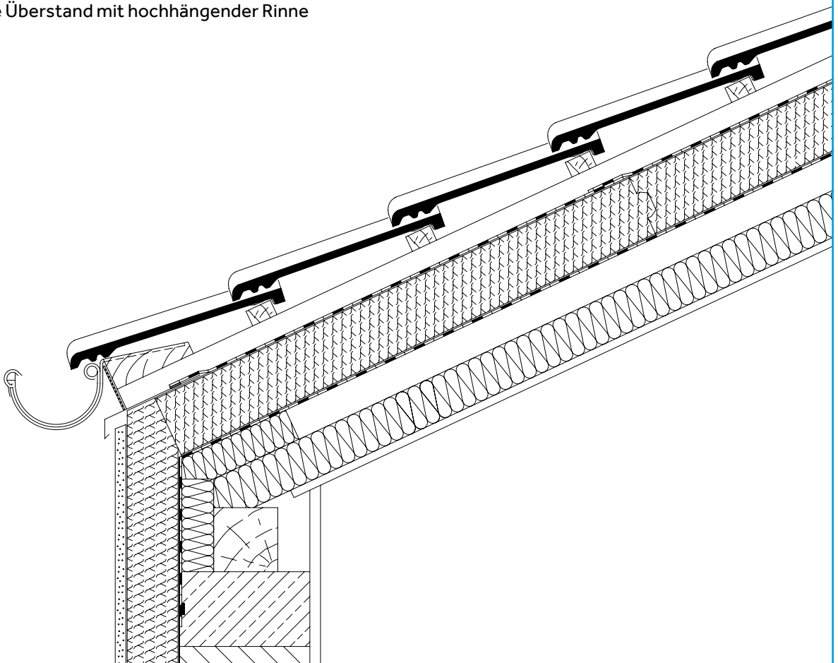
Traufe ohne Überstand mit hochhängender Rinne
