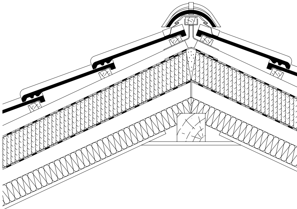
First mit zweiseitigem V-Schnitt
