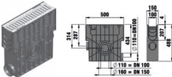
Einlaufkasten mit Kunststoff-Eimer, mit Klemm-Stegrost, Pkw-befahrbar, arretiert
