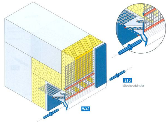
maxit Abschlussprofil mit Tropfkante
