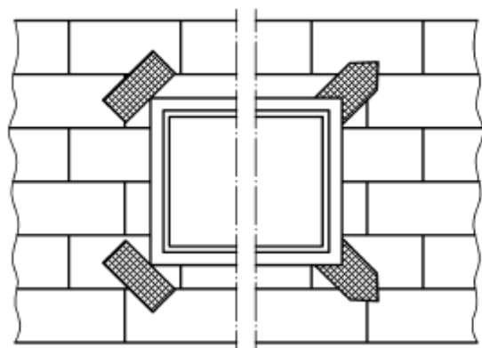
Ausführungsbeispiele Diagonalarmierung
