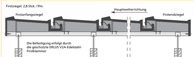
Firstlüfterziegel Nr. 19 Lü
