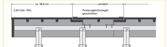
Firstziegel Nr. 15
