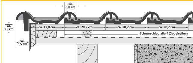
Linker Ortgang*
