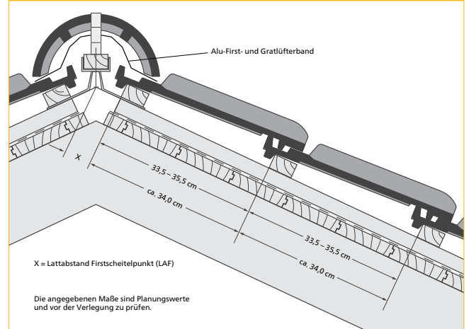
Firstziegel Nr. 15 mit Standardziegeln
