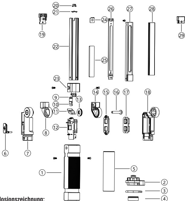
Explosionszeichnung:
