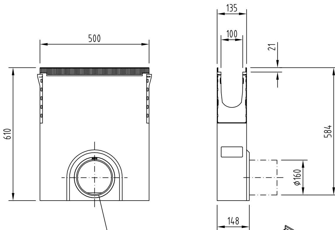
Lippenlabyrinth-Dichtung DN/OD 160
