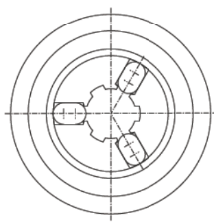
Ringverschluss Typ C
