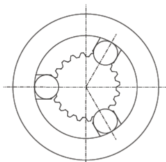
Ringverschluss Typ D1
