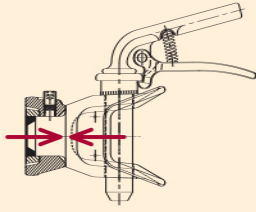
Nicht selbsttätige Kupplungen
