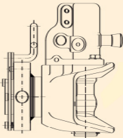
Kuppelbolzen Verschleißgrenzen
