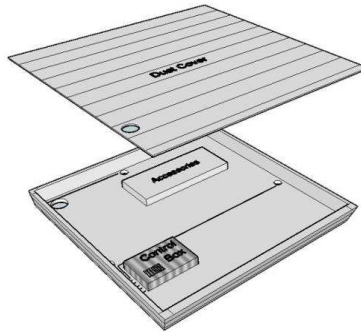
Bild G4: Entfernen Sie die Staubabdeckung
