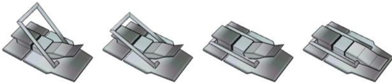
Abbildung 1 Äußeres Klickverschlussverfahren
