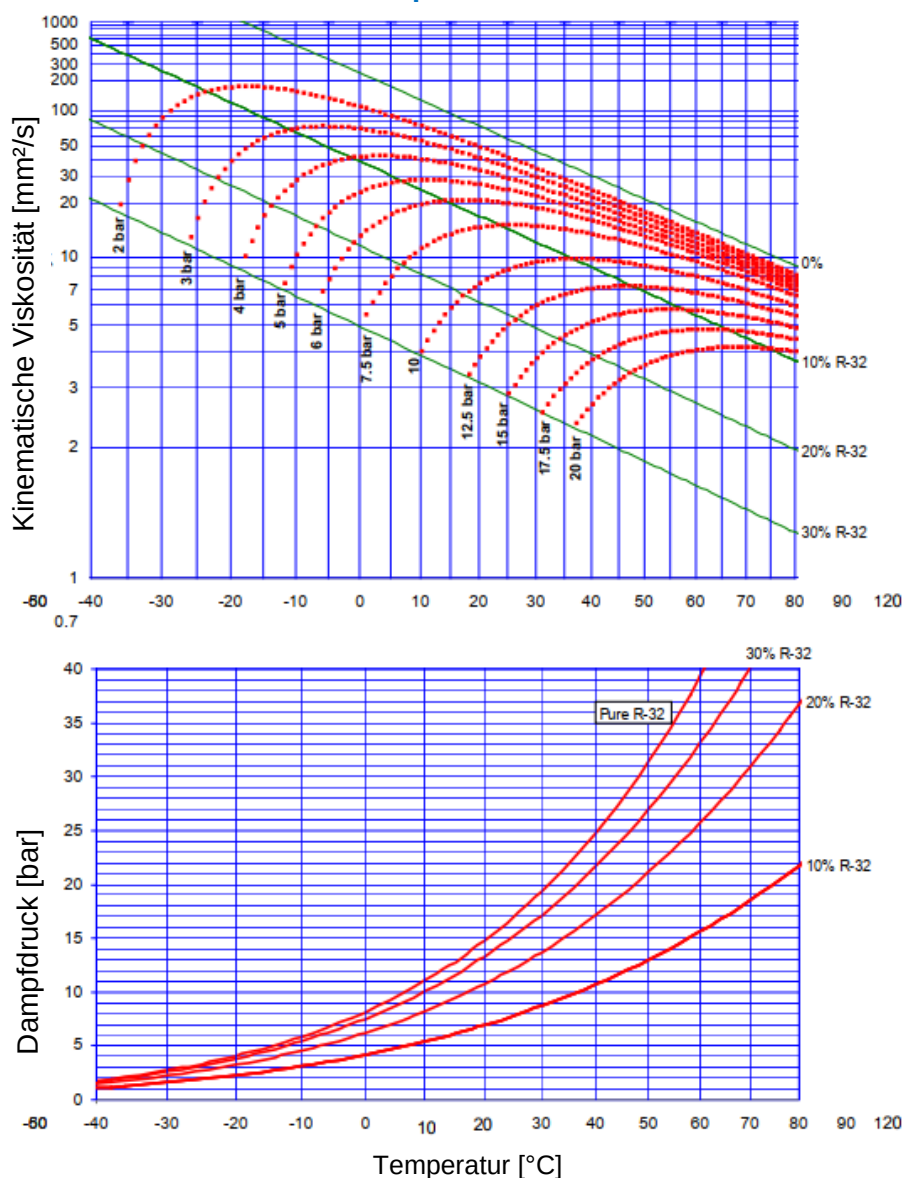
Kinematische Viskosität und Dampfdruck: RENISO TRITON SEZ 32 und R32
