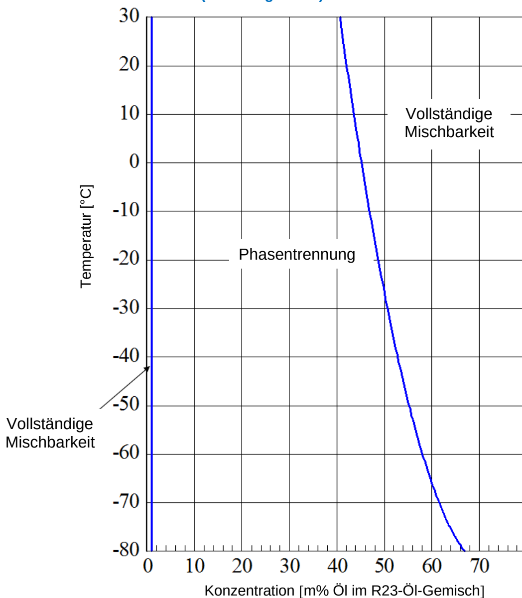
Kältemittelmischbarkeit (Mischungslücke): RENISO TRITON SEZ 32 und R23
