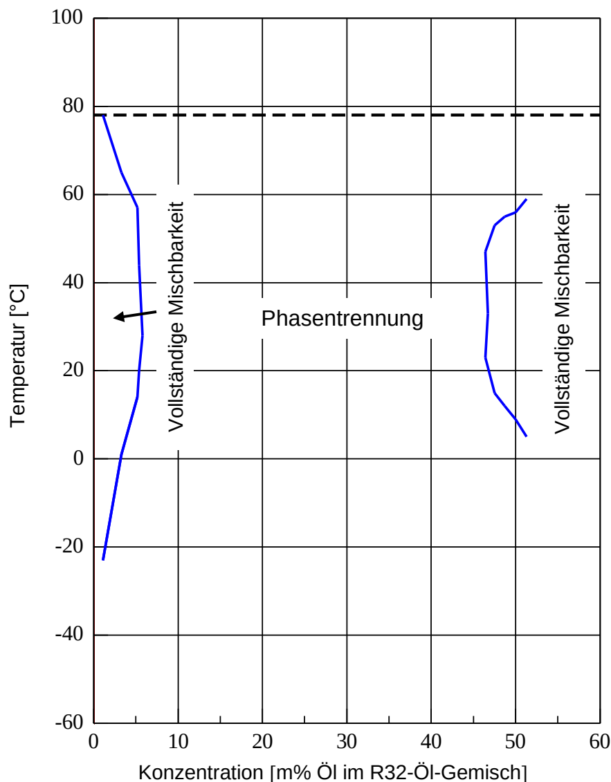
Kältemittelmischbarkeit (Mischungslücke): RENISO TRITON SEZ 32 und R32
