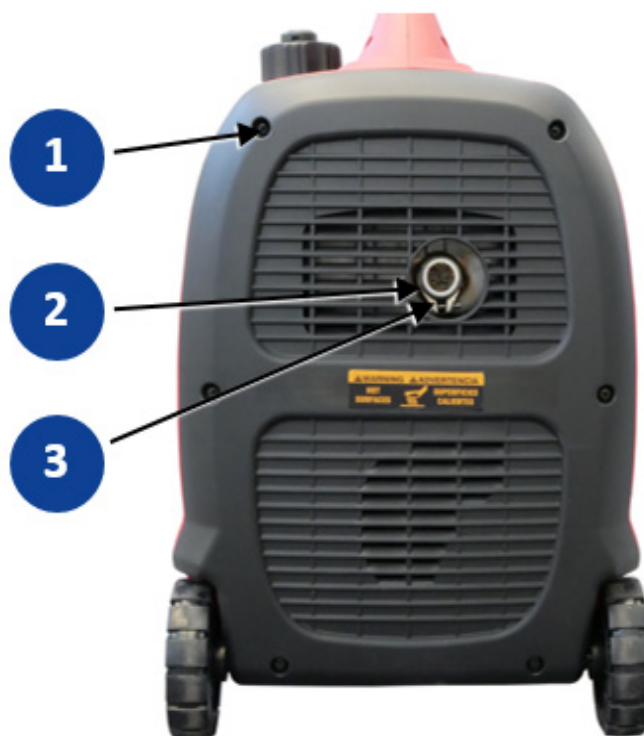
Abb. 8-7 Funkensieb
