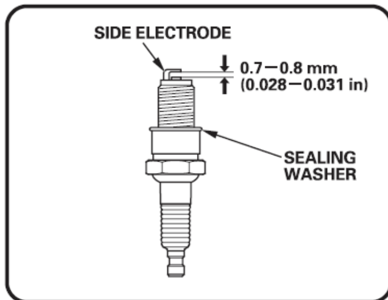
Abb. 8-6 Zündkerze prüfen
