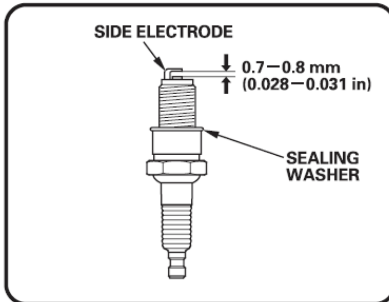
Abb. 9-8 Zündkerze prüfen
