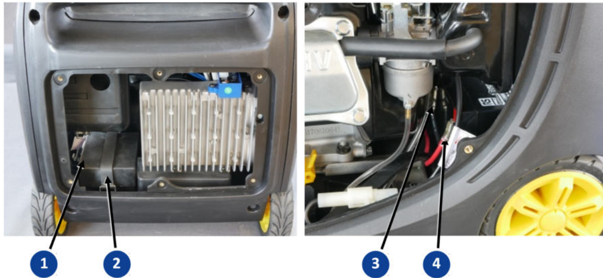
Abb. 9-9 Starterbatterie wechseln
