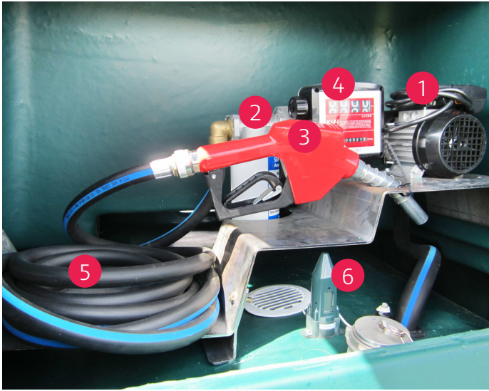
Modell DFD (Pumpe in abschließbarem Pumpenschrank)
