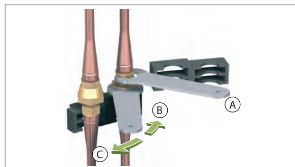
Abb. 15: Abschrauben der rechten Überwurfmutter
