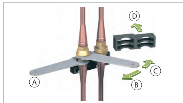
Abb. 14: Abschrauben der linken Überwurfmutter
