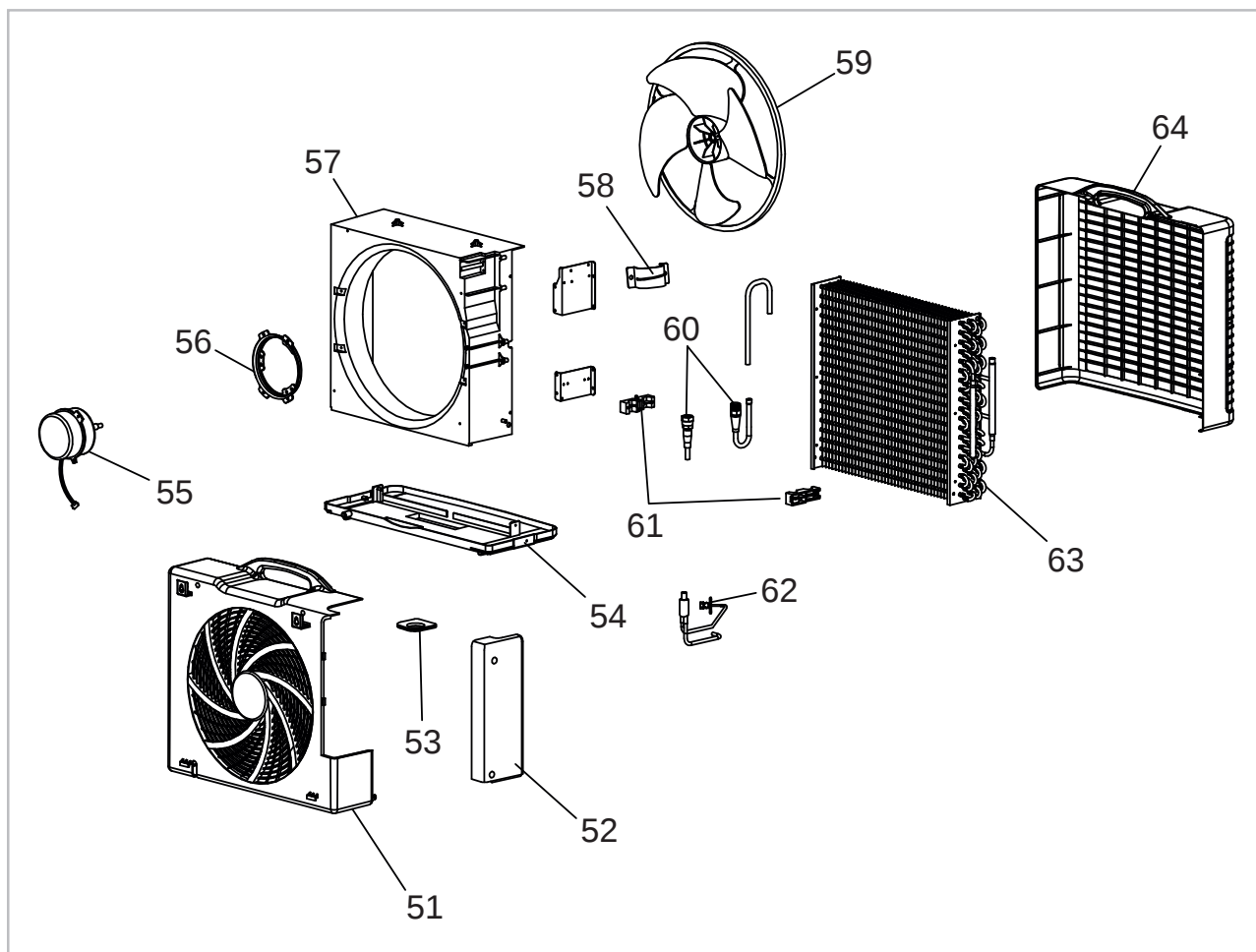
Abb. 19: Explosionszeichnung Außenteil
