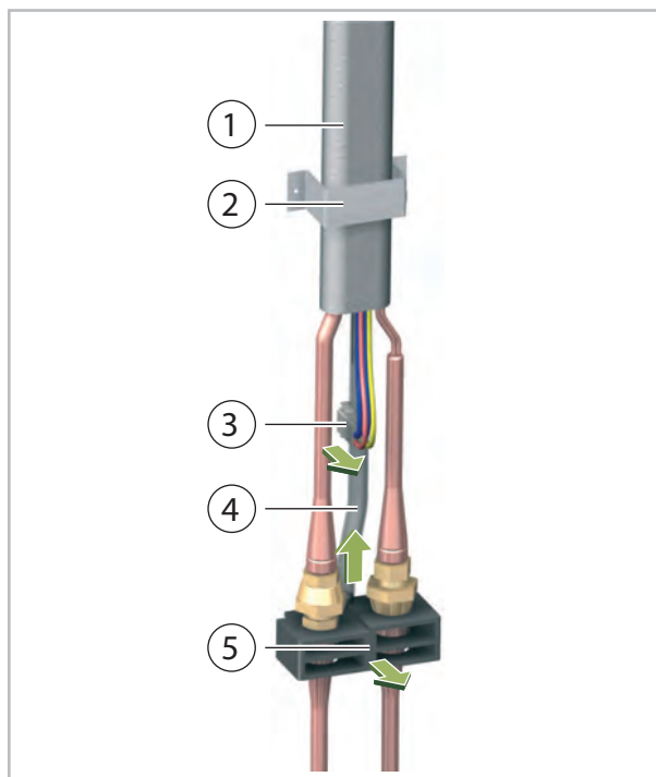
Abb. 13: Demontage Verbindungsleitung
