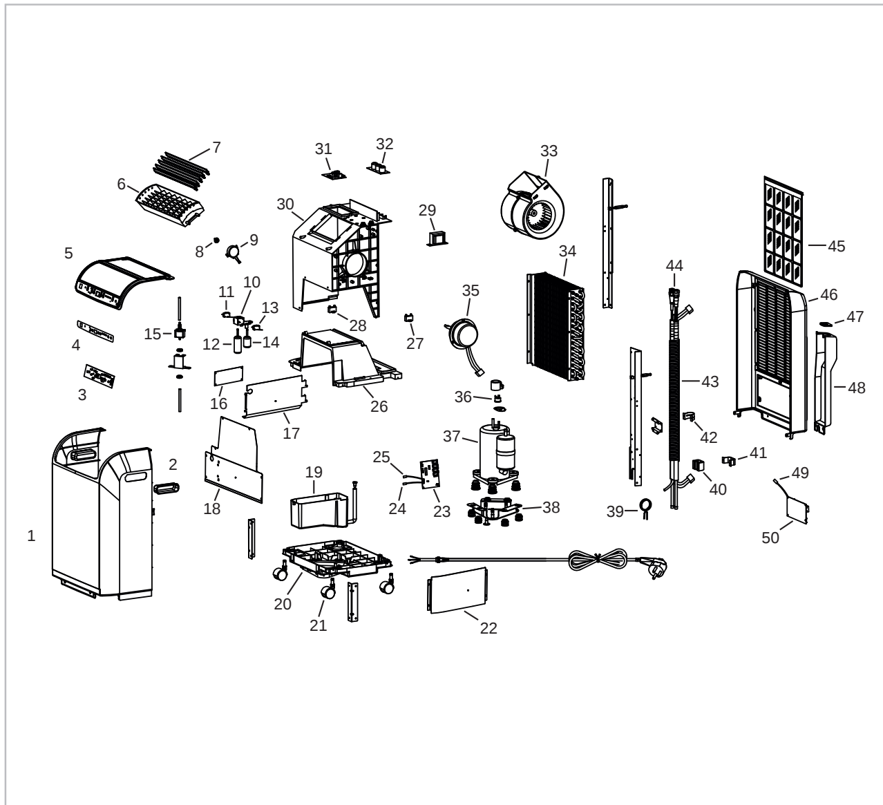
Abb. 18: Explosionszeichnung Innengerät
