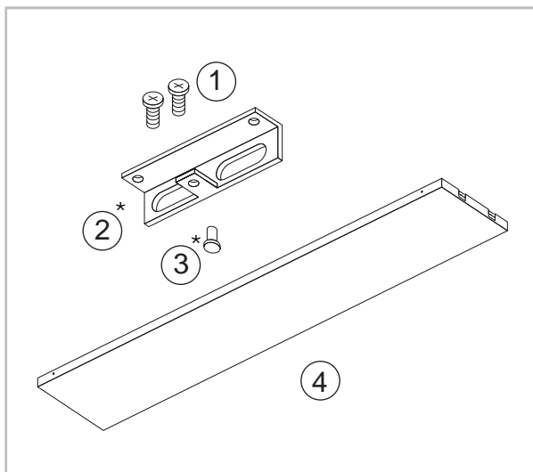
Abb. 2: Lieferumfang
