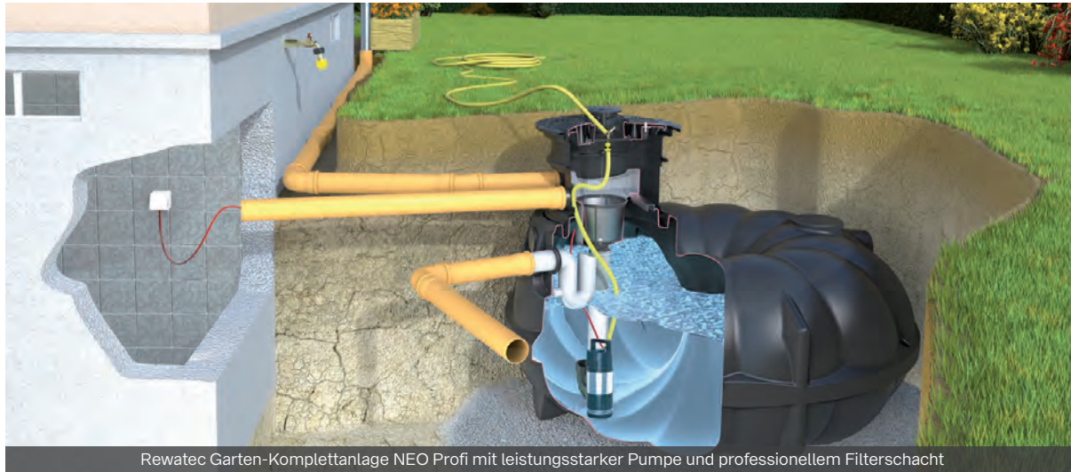
Rewatec Garten-Komplettanlage NEO Profi mit leistungsstarker Pumpe und professionellem Filterschacht
