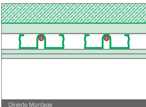
Direkte Montage
