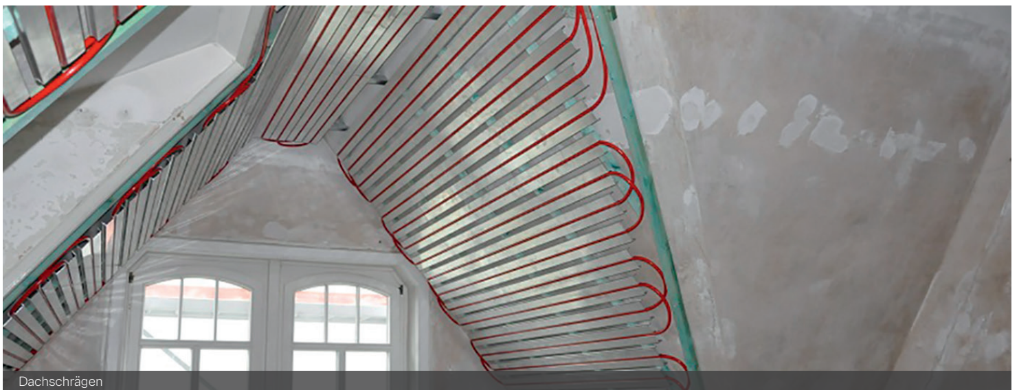
Dachschrägen
