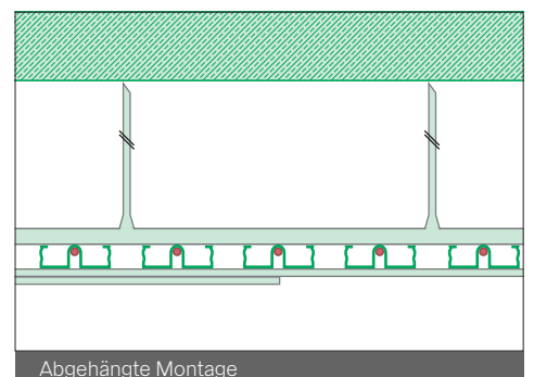
Abgehängte Montage
