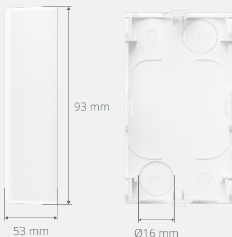
Monteringsdel med skruvhål samt Ø16 mm slang
