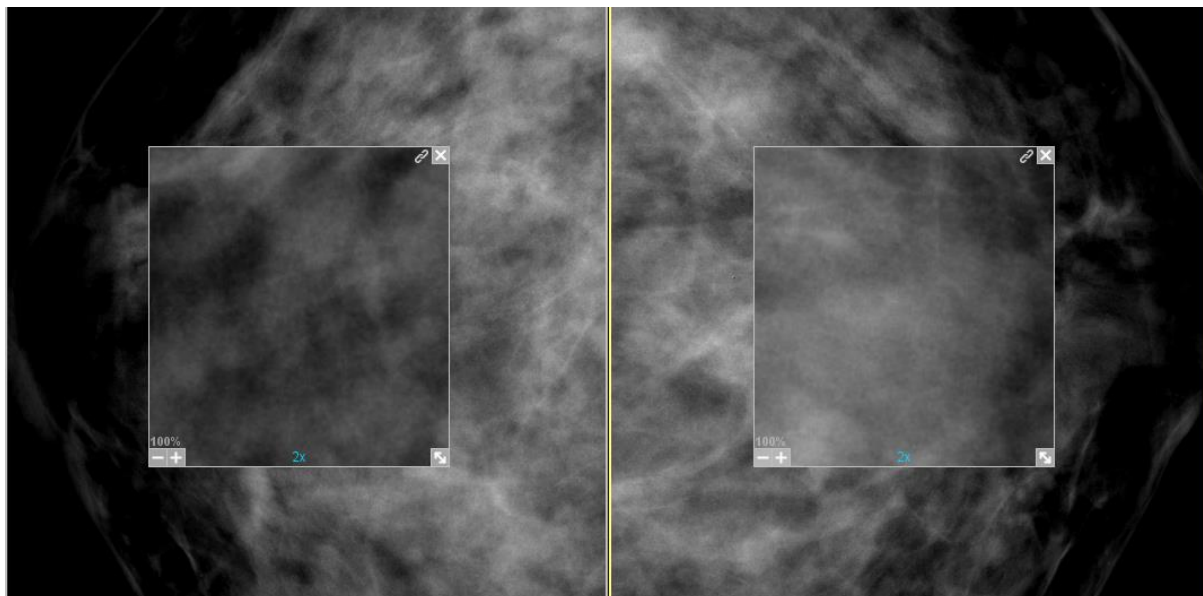
Figure 22 : Loupes synchronisées
