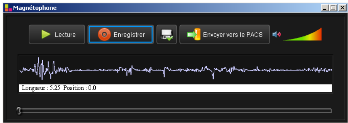
Figure 30 : Magnétophone interne
