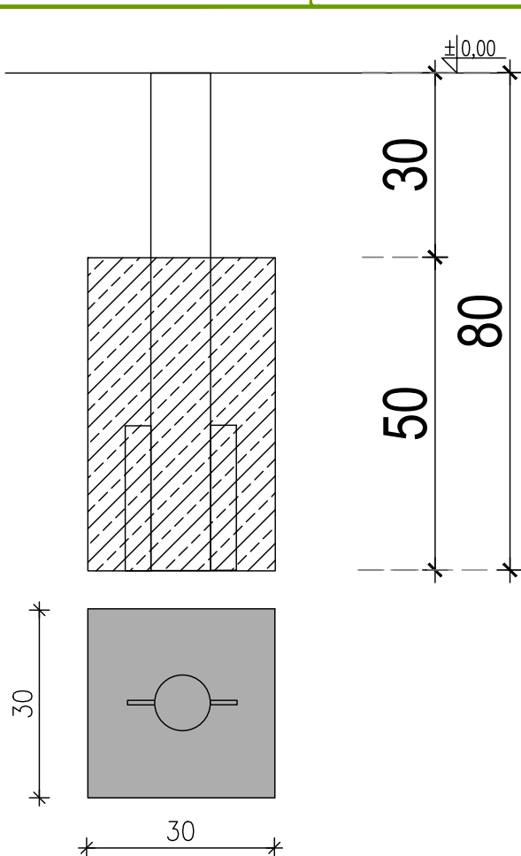
BW-F-01: WYMIARY (szer x dł x wys): 30x30x50 cm WAGA: xxx kg BETON: C16/20
