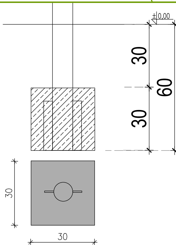
BW-F-01: WYMIARY (szer x dł x wys): 30x30x30 cm WAGA: xxx kg BETON: C16/20
