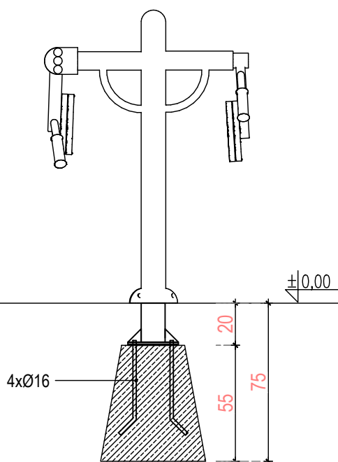
WARIANT 1 - FUNDAMENT PREFABRYKOWANY
