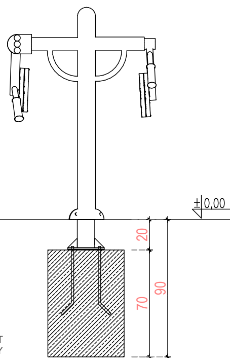
WARIANT 2 - FUNDAMENT WYLEWANY
