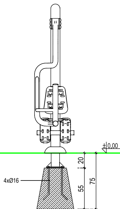
WARIANT 1 -FUNDAMENT PREFABRYKOWANY
