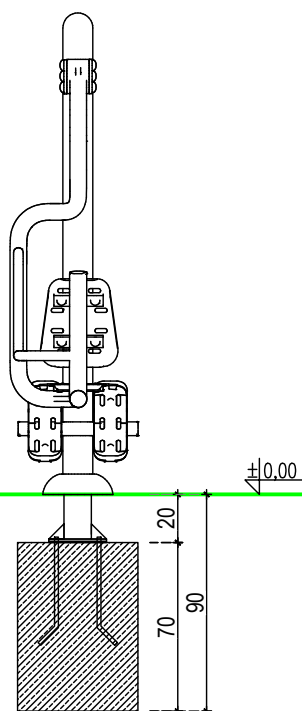
WARIANT 2 -FUNDAMENT WYLEWANY
